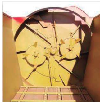
TURBINA PROFESIONAL DOBLE TRITURADOR Y DOBLE CUCHILLA DE ACERO PARA PRODUCTOS MUY COMPACTOS O CON MUCHA PAJA
